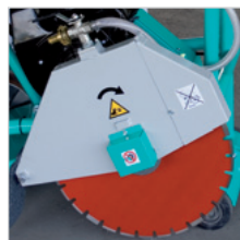
Carter disco con parte anteriore sollevabile
